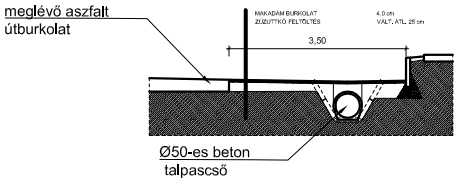
TERVEZETT ÁLTALÁNOS METSZET M = 1 : 50
